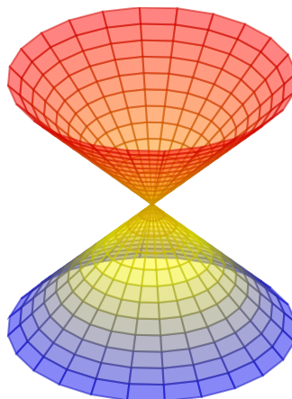
Infinite cone
